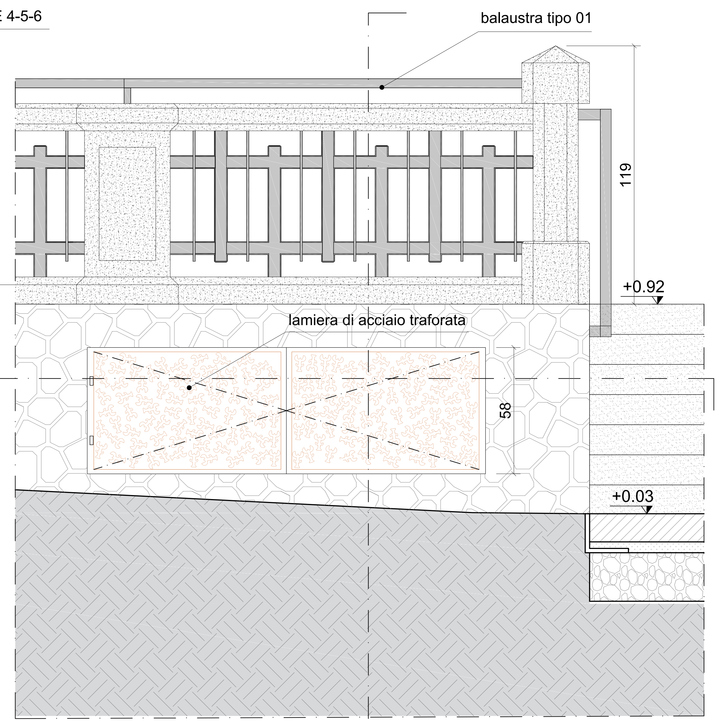
SEZIONE B-B
