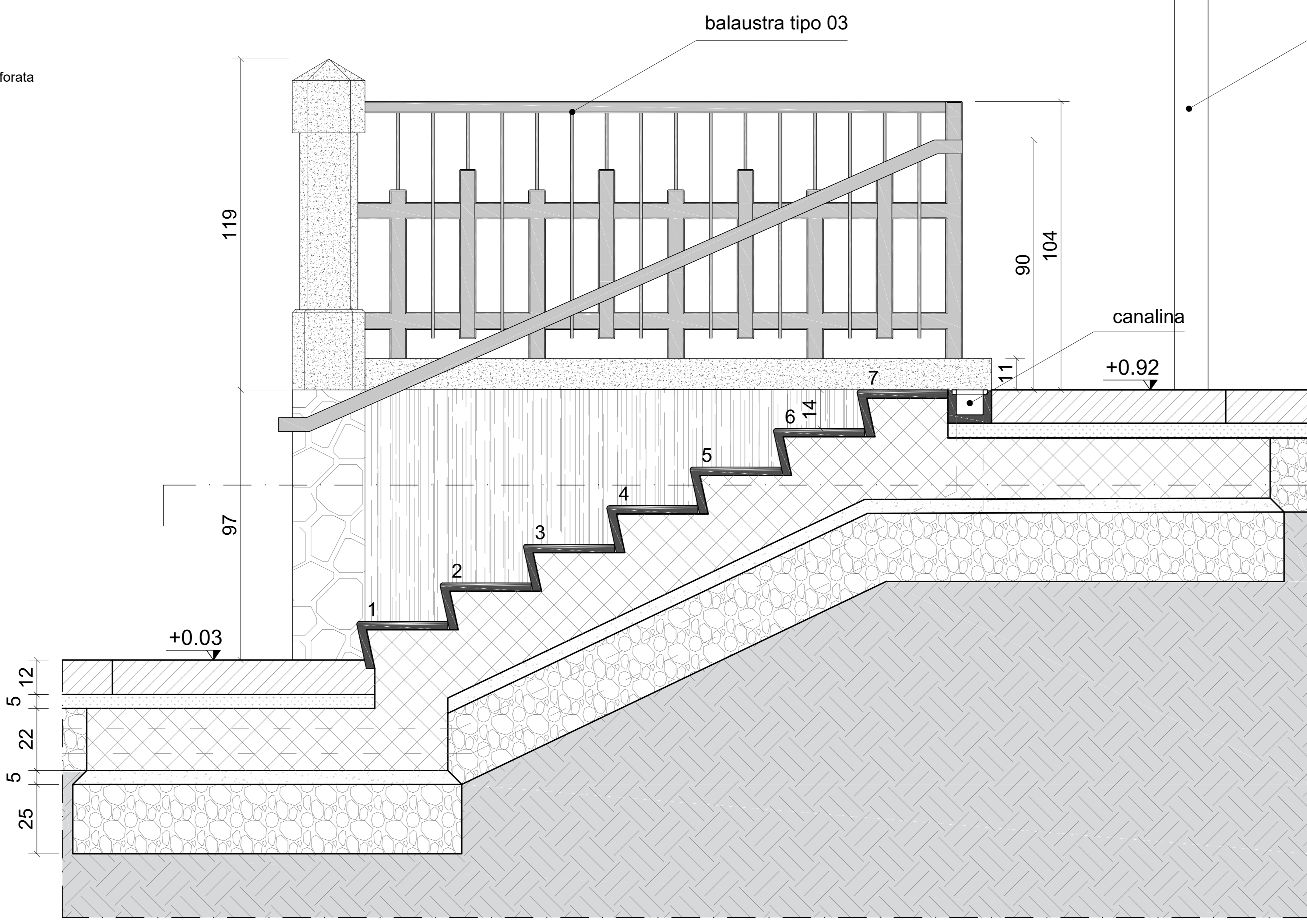
SEZIONE A-A
