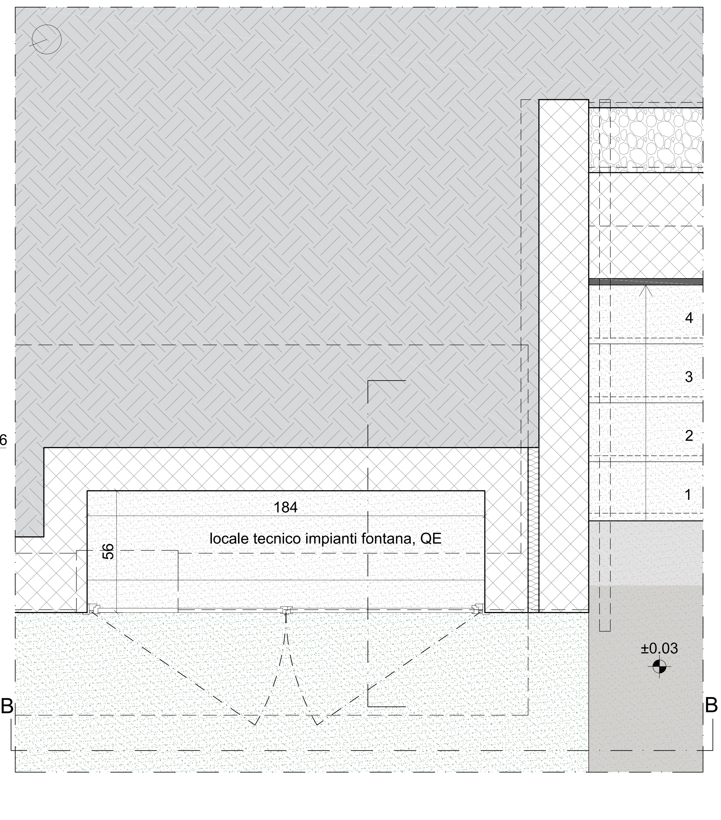
SEZIONE B-B
